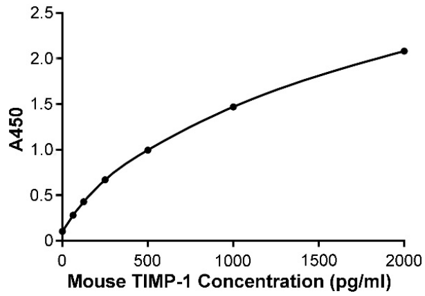
图3. Mouse TIMP-1 ELISA Kit的标准曲线。实测数据会因实验条件、检测仪器等的不同而存在差异，图中数据仅供参考。
